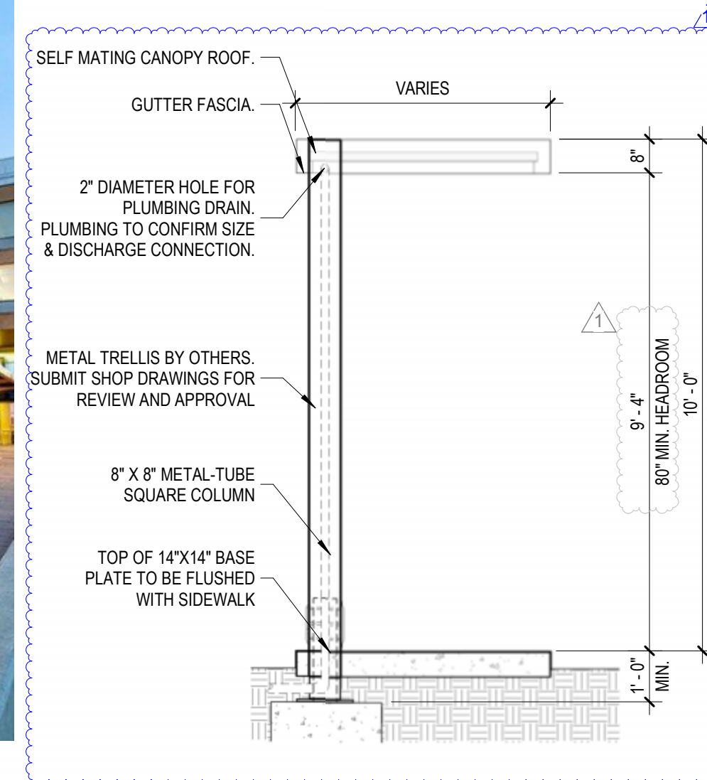
7 TRELLIS DETAIL SECTION SCALE: 3/8" = 1'-0"
